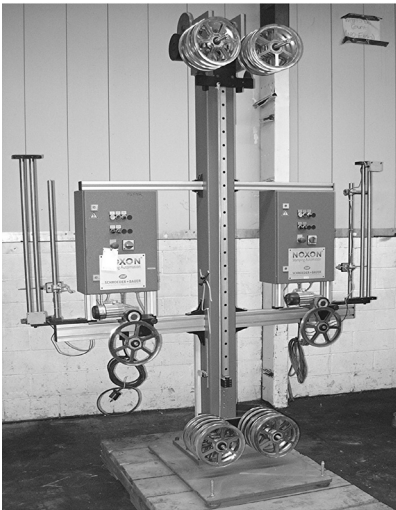
Noxon/Schroeder & Bauer Precision Press Accumulator
